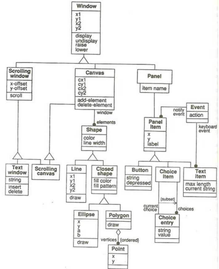
OMT (Object Modeling Technique)
