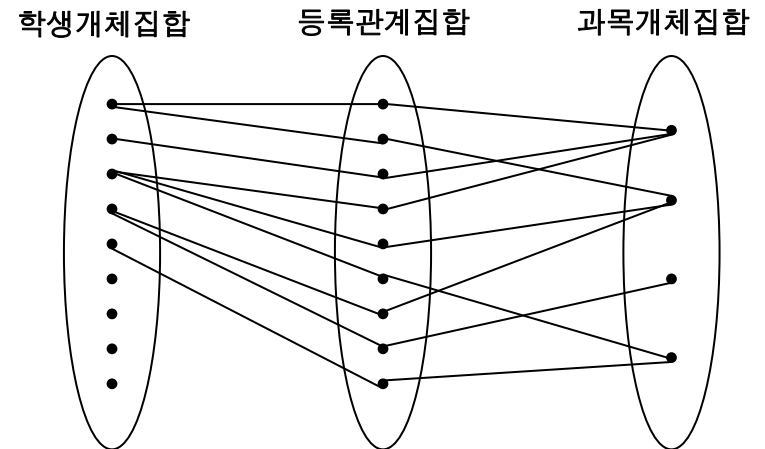
등록 관계 인스턴스
