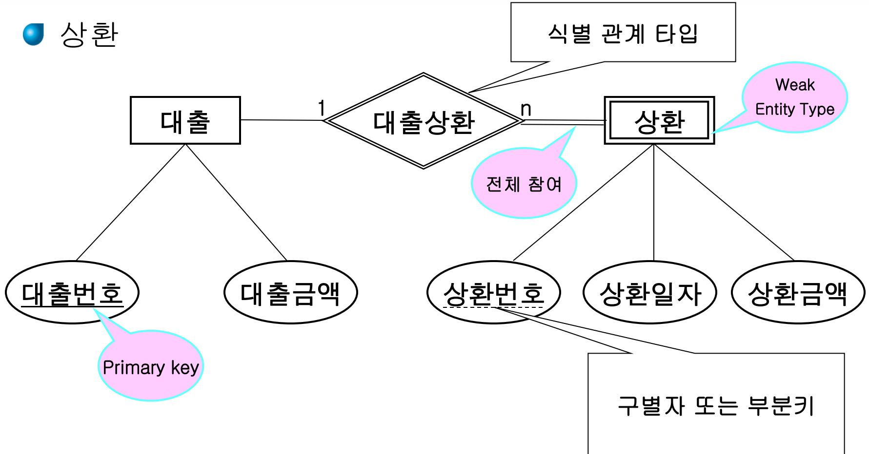
대출 상환 관계의 E-R 다이어그램
