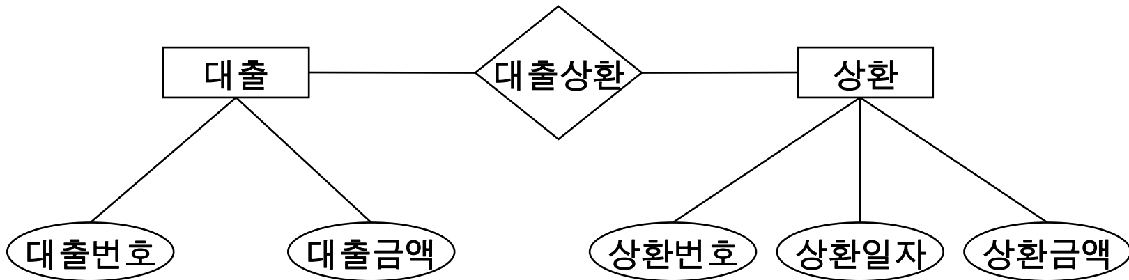
대출 상환 관계 ( 주 개체: 대출, 종속 개체: 상환)
